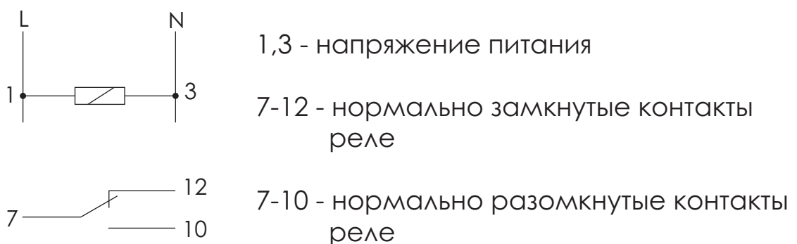
Рис.2 Назначение контактов.
