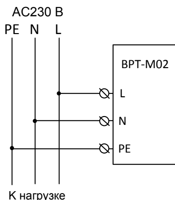
Схема подключения для трёхпроводной сети
