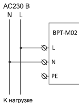
Схема подключения для двухпроводной сети
